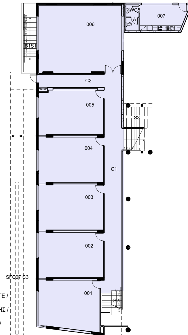
ΕΠΙΠΕΔΟ +139,60 ΗΜΙΥΠΟΓΕΙΟ ΣΥΝΟΛΙΚΟ ΕΜΒΑΔΟΝ 392,93m 2
